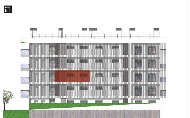
Alçado Poente 1:100
