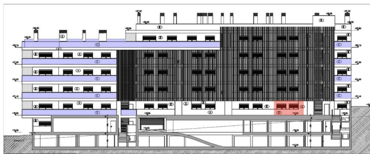
ALÇADO POENTE
